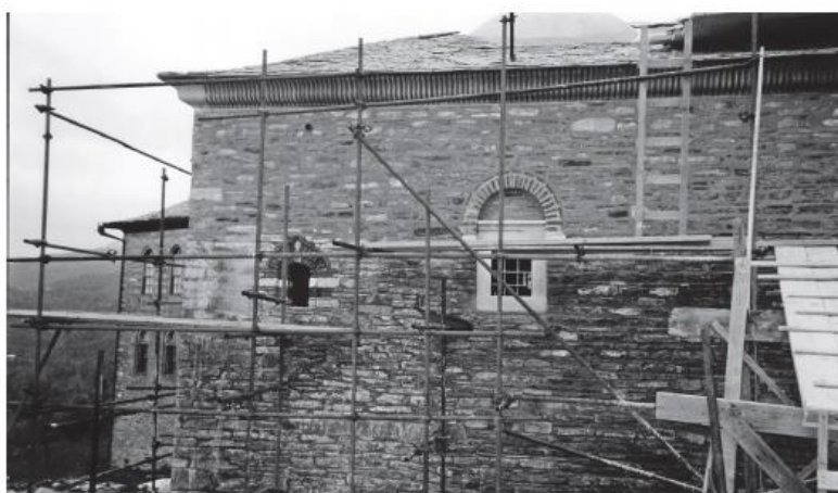
Είκ. 27. Βόρεια ὄψη μετά τὸ πέρασ τῶν ἐργασιῶν.
